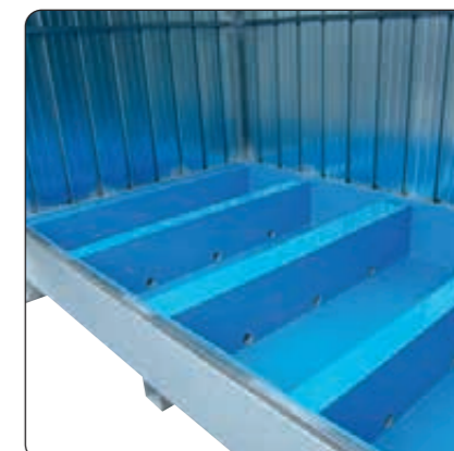
Vasca supplementare in polipropilene sp. 5 m/m, saldata e testata per assicurare la tenuta e la corrosione, a garanzia di eventuali sversamenti accidentali di acidi con concentrazioni elevate, da integrare all'interno della vasca metallica di contenimento.
