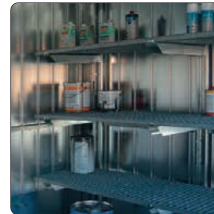
Scaffalatura modulare costituita da piani regolabili in altezza in grigliato zincato. N. livelli: 3 di profondità 500 mm
