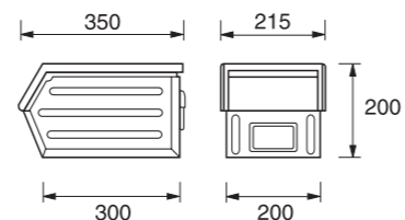
DIMENSIONI DIMENSION 350x200x200 h. CAPACITA' CAPACITY LT. 12,5
