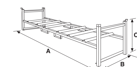
SPF 373 Per 3 fusti da 200 litri For 3 x 200 litre drums
