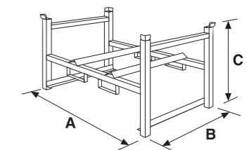
SPF 351 Per 1 fusto da 200 litri For 1 x 200 litre drum
